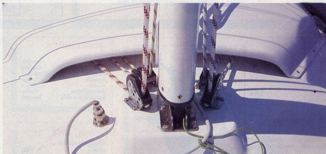
L'albero a doppio ordine di crocette aguartierate che poggia in coperta, elimina il rischio di infiltrazioni d'acqua e semplifica le operazioni di montaggio. Le drizze corrono sotto una calandra in vetroresina fissata con viti autofilettanti, così da facilitarne l'ispezione. In questa zona lo spazio prendisole è comunque limitato.
